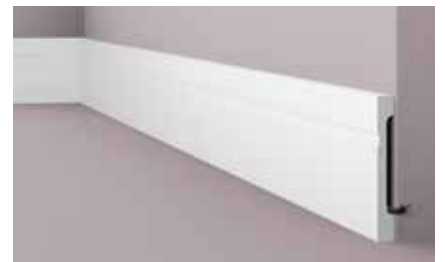
FD15 WALLSTYL® 150 x 18 x 2000 mm
