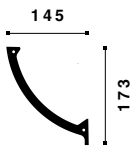
L3 ARSTYL® 173 x 145 x 2000 mm
