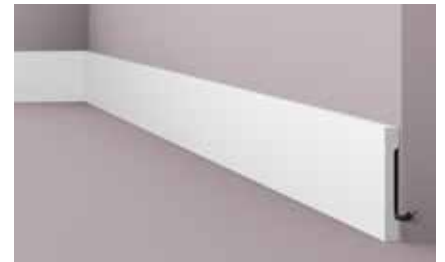
FD2S WALLSTYL® 110 x 15 x 2000 mm
