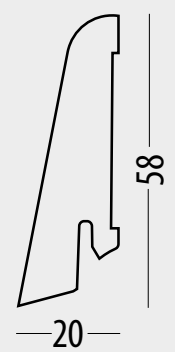
Länge: 2400 mm Höhe: 58 mm Tiefe: 20 mm
