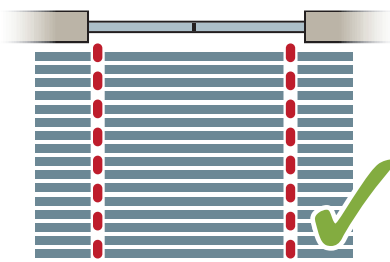
Korrekte Teilung bei Stablängen über 3000 mm bzw. über 60 kg Gewicht.
